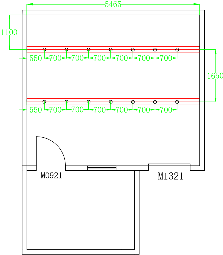
槽钢安装示意图
